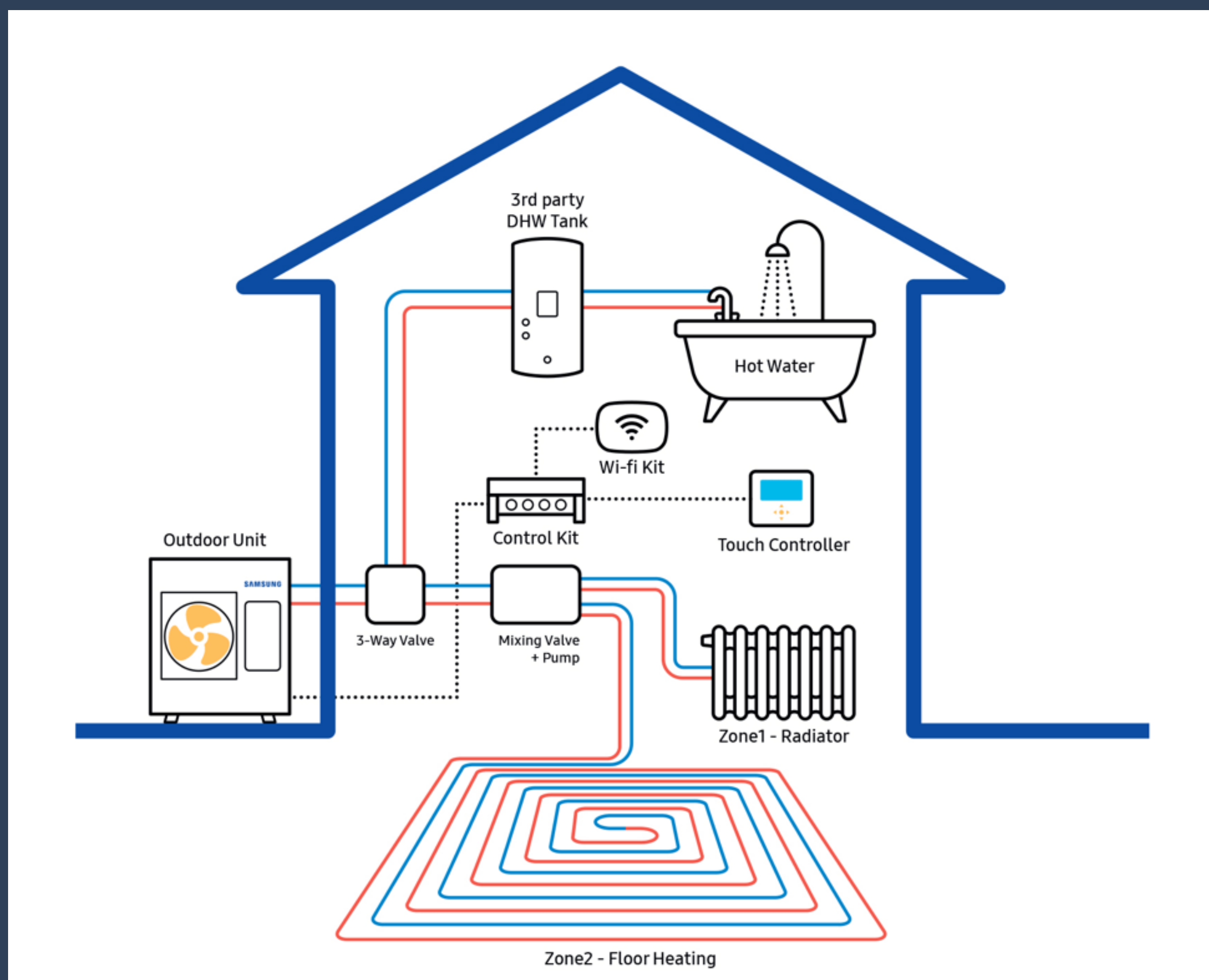
RYS. 5 - OGÓLNY SCHEMAT INSTALACJI Z POMPĄ CIEPŁĄ.
