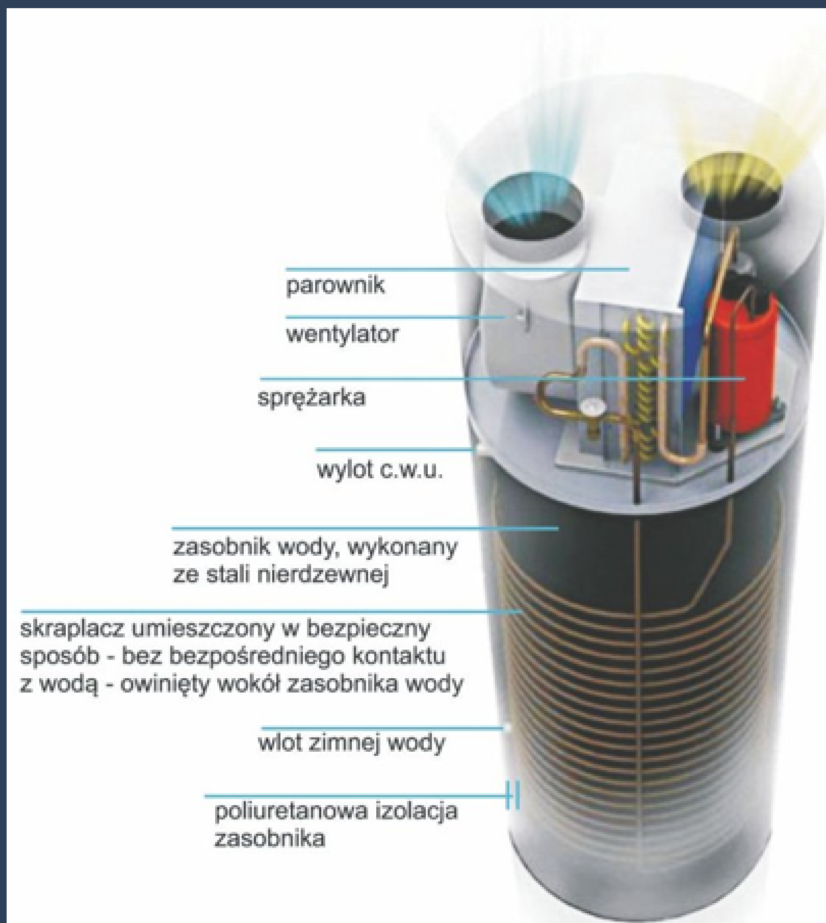
RYS. 7 - KOMPAKTOWA POMPA CIEPŁA DO C.W.U.
