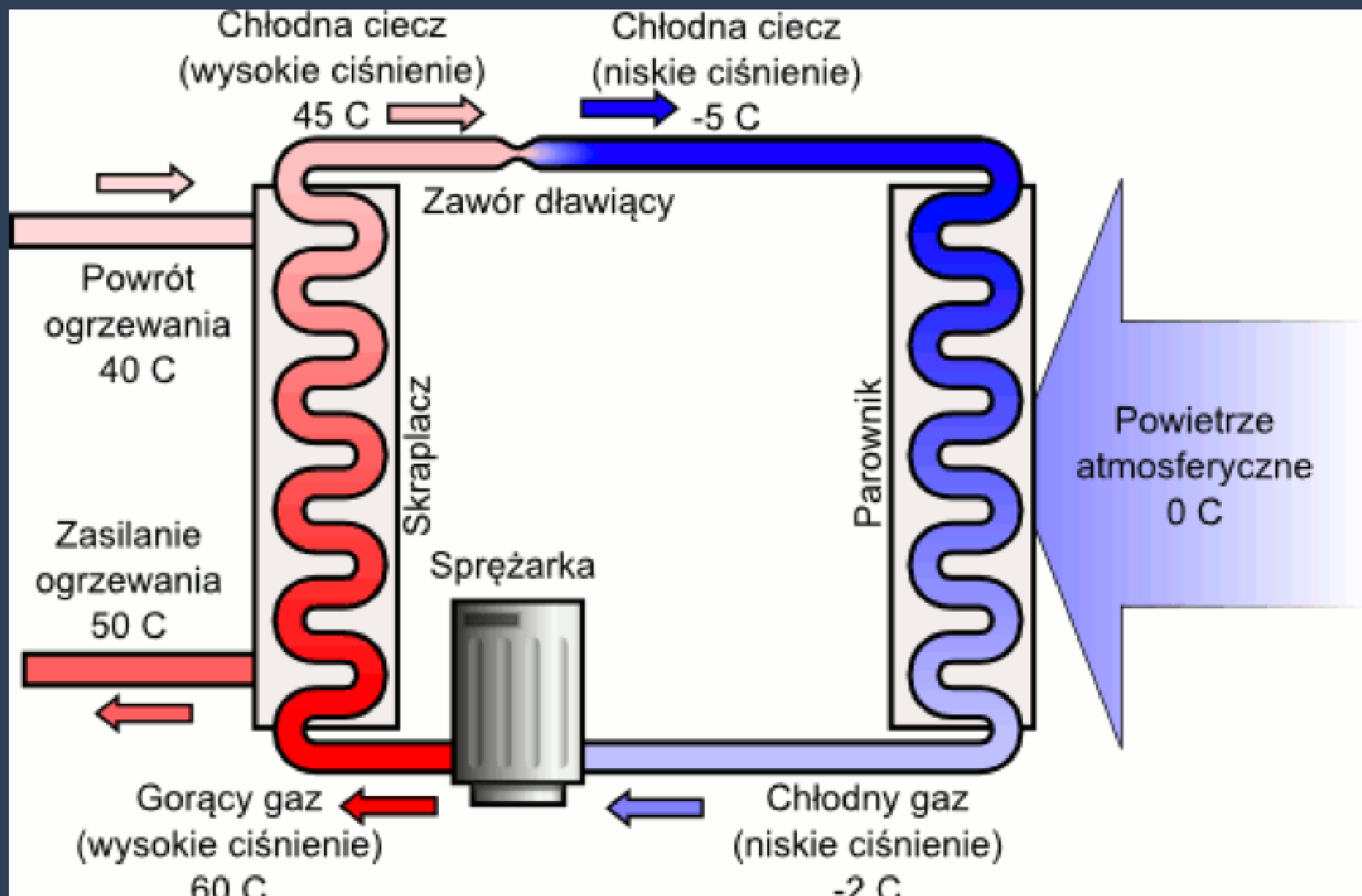
RYS. 4 - OGÓLNY SCHEMAT UKŁADU POMPY CIEPŁA.
