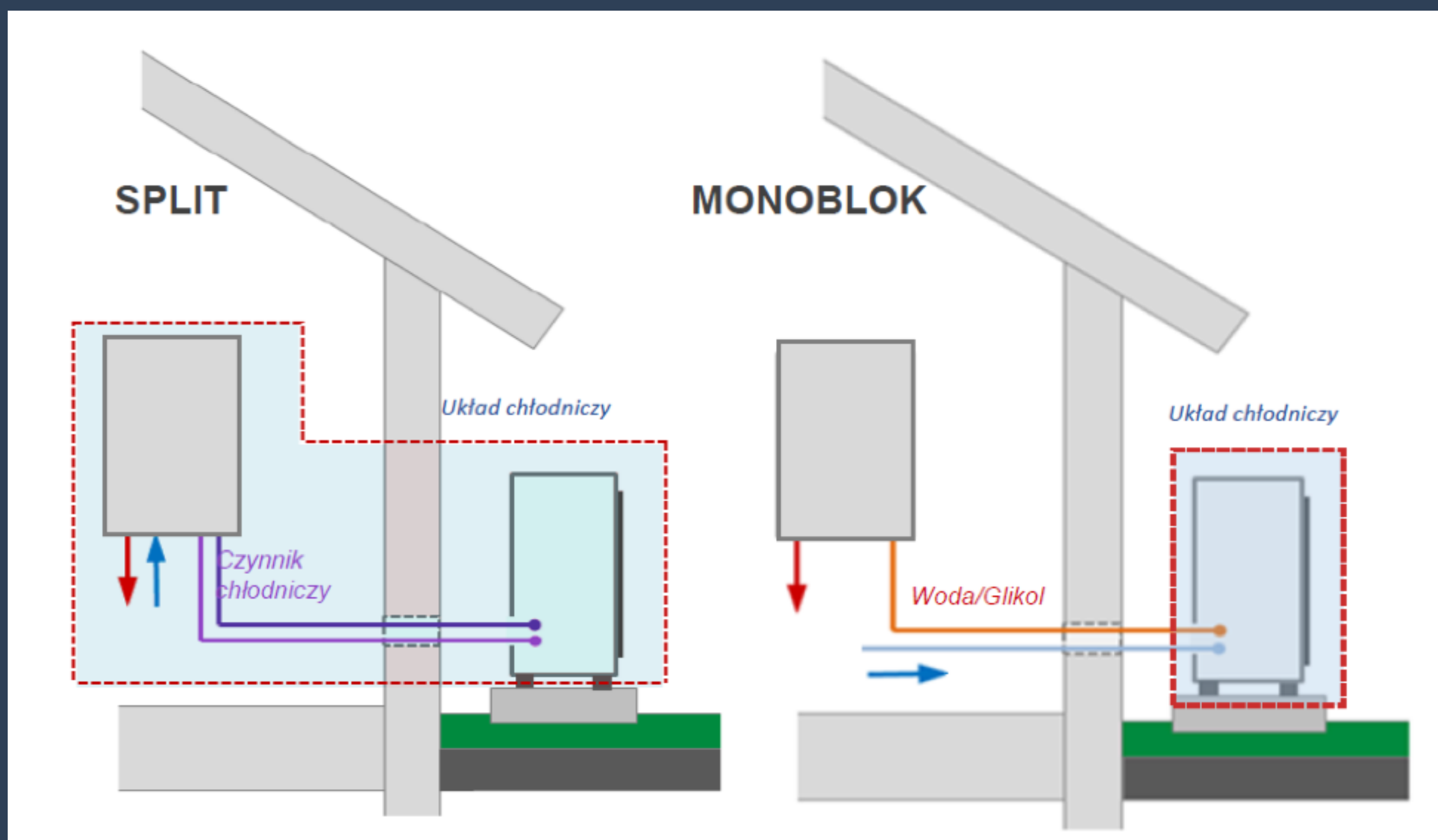
RYS. 6 - PO LEWEJ WERSJA POMPY CIEPŁA SPLIT, PO PRAWEJ MONOBLOK.
