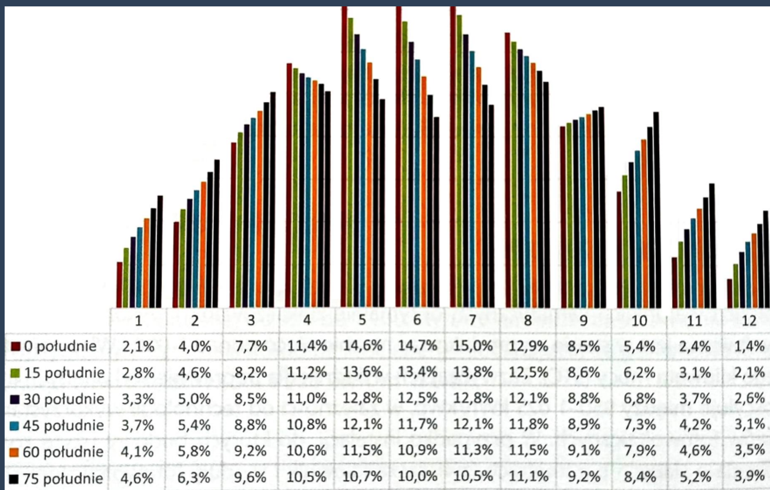
RYS. 3 - UZYSK PROCENTOWY W ZALEŻNOŚCI OD KĄTA NACHYLENIA MODUŁÓW FOTOWOLTAICZNYCH DLA KAŻDEGO MIESIĄCA W SKALI ROKU.
