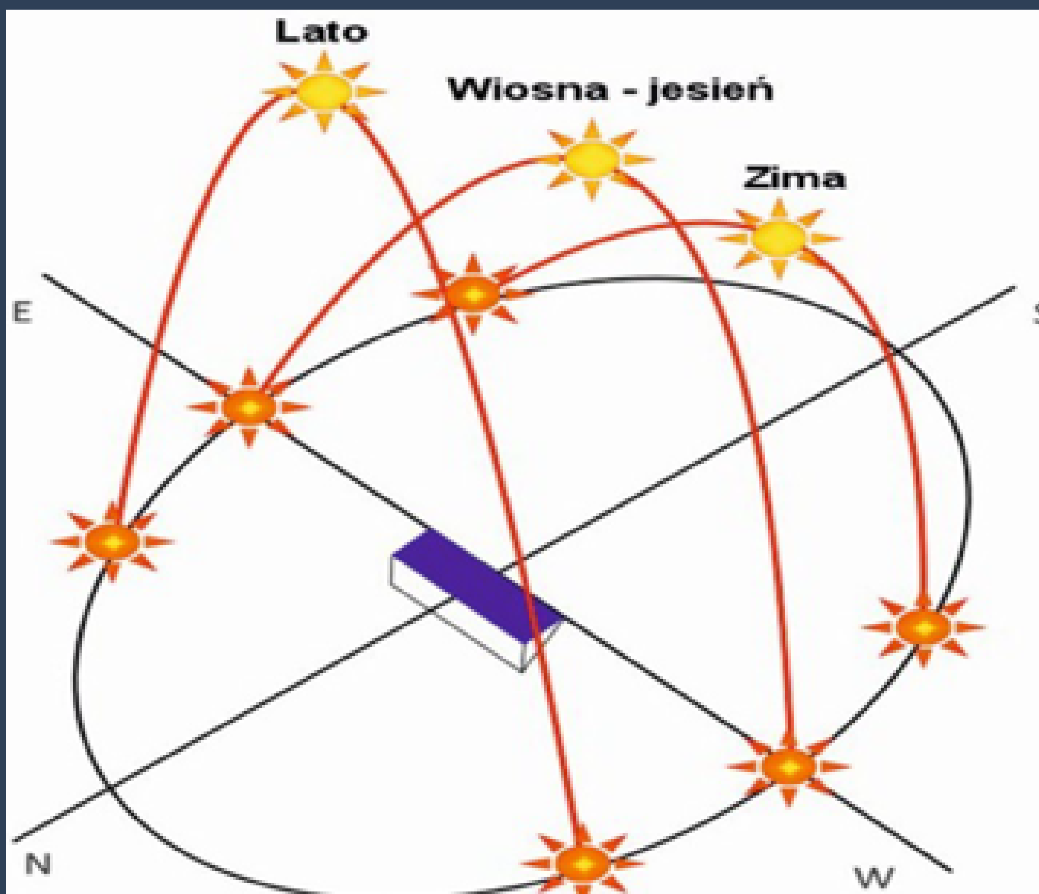
RYS. 2 - WYSOKOŚĆ SŁOŃCA W POSZCZEGÓLNYCH PORACH ROKU.
